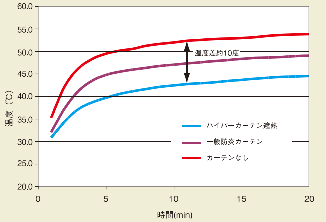
遮熱効果測定結果
